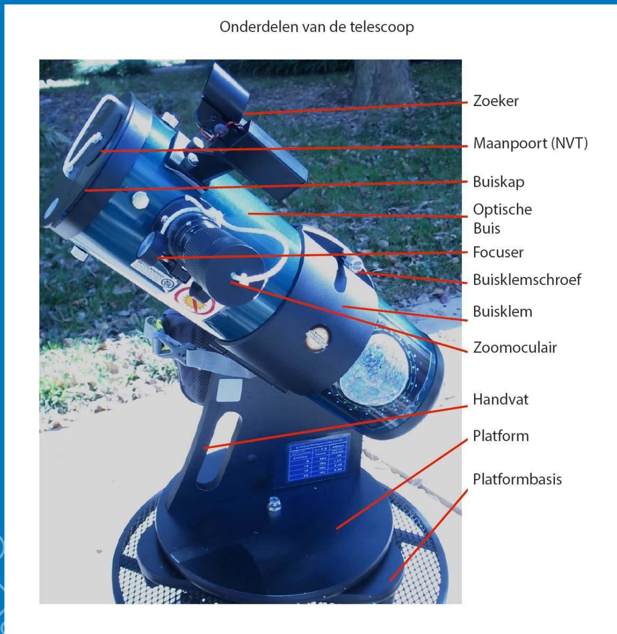
Afbeelding 3: De onderdelen van de telescoop
